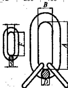
Звено типа Т
