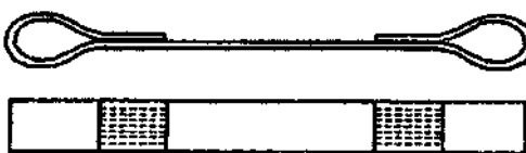
Рис. 1. Одиночный петлевой строп с мягкими плоскими петлями
