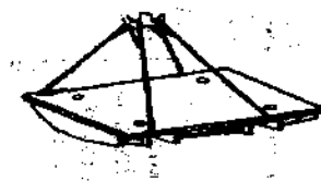
Схема строповки рамы тележки
